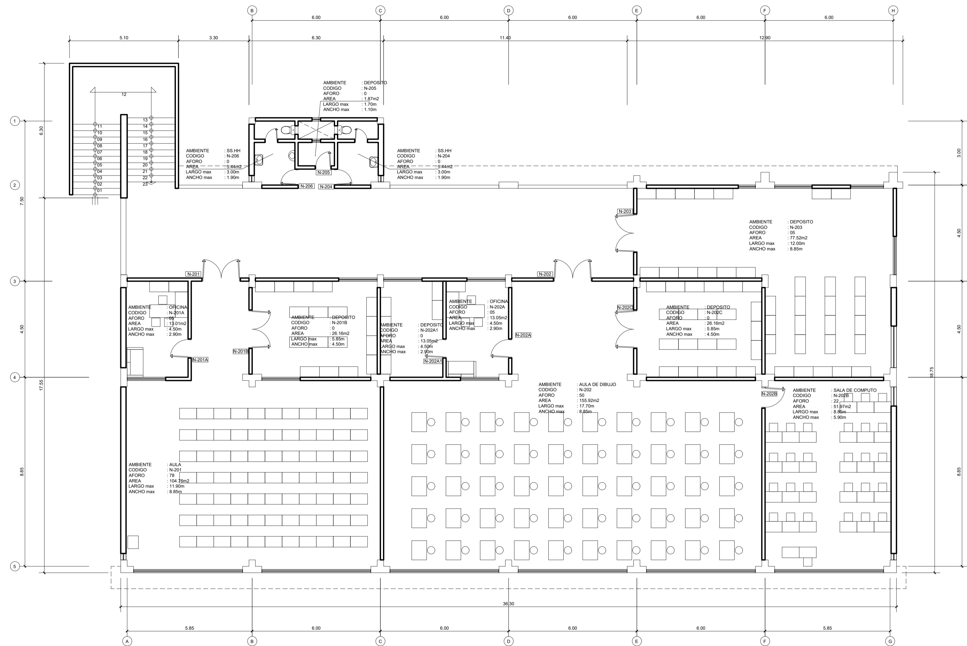
SEGUNDA PLANTA AREA TECHADA = 709.88m 2 AFORO = 165 ESCALA 1:100
